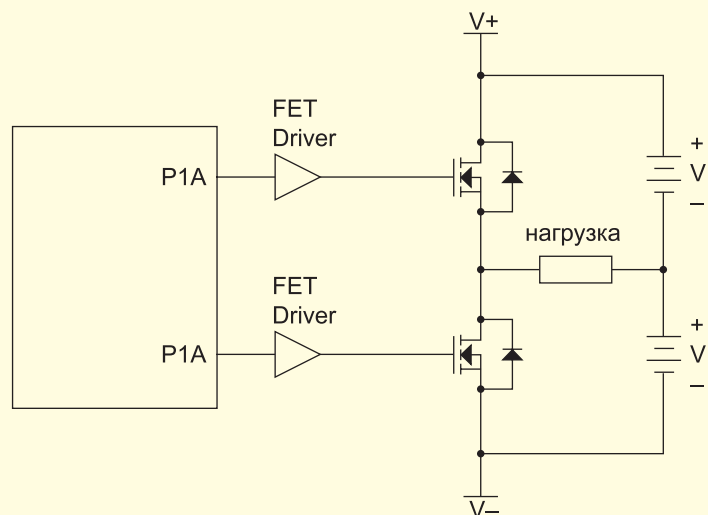
Рисунок 2 Включение модуля ЕССР в режиме «полумост»
