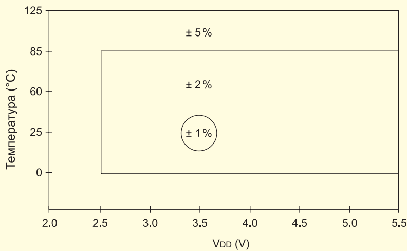
Рисунок 1 Низкая погрешность RC генератора во многих приложениях позволяет отказаться от кварца
