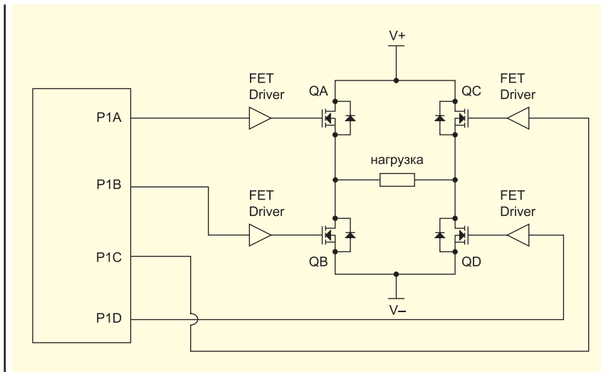
Рисунок 3 Включение модуля ECCP в режиме «мост»
